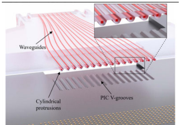
Edge Coupling FAU
