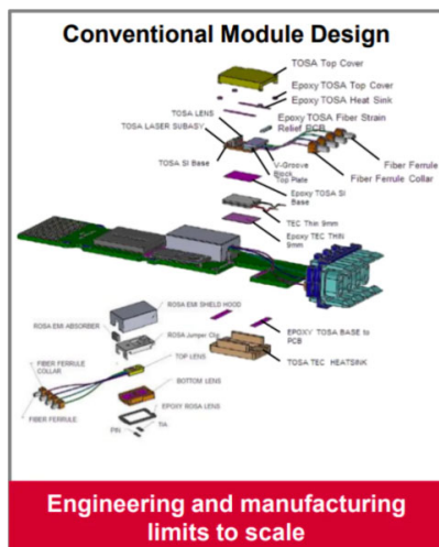
EML收發器
