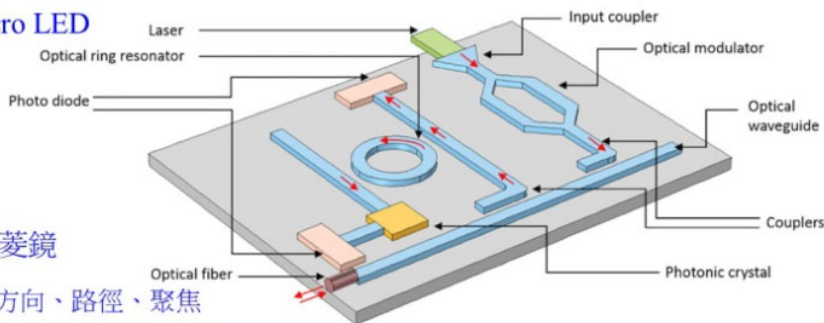
PIC內部元件示意圖
