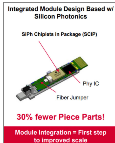
矽光收發器
